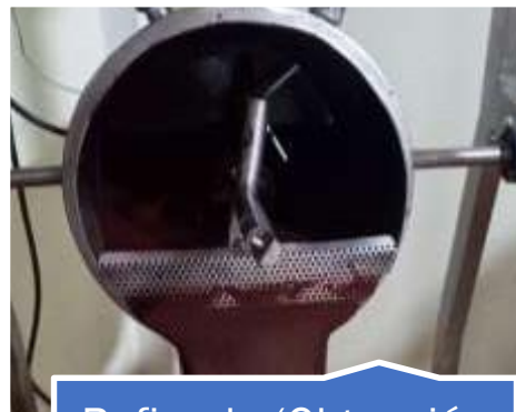
Refinado (Obtención de licor de cacao)
