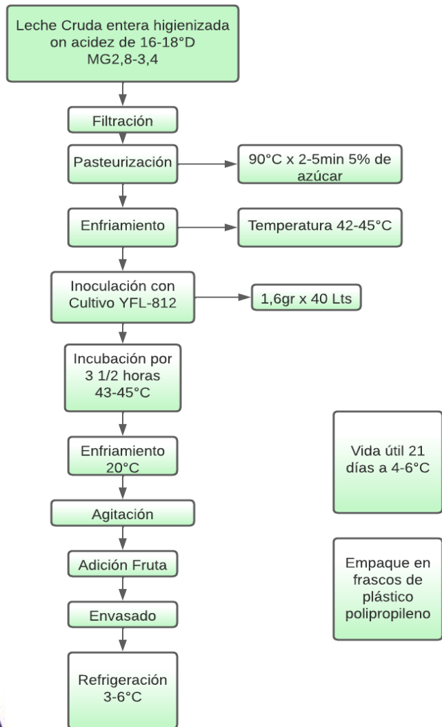
PROCESO DE FABRICACION DE YOGURT BEBIBLE
